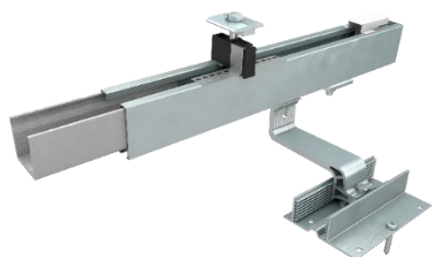
EASY ROOF TOP pour tuiles galbées. Éléments de fixation et rail en aluminium. Visserie en inox.
